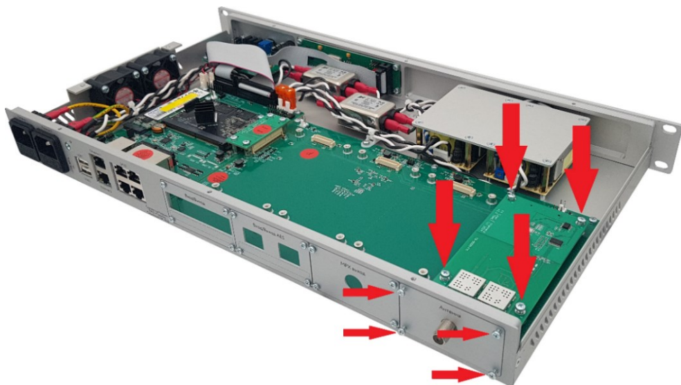
Рисунок 10 – Установка модуля
