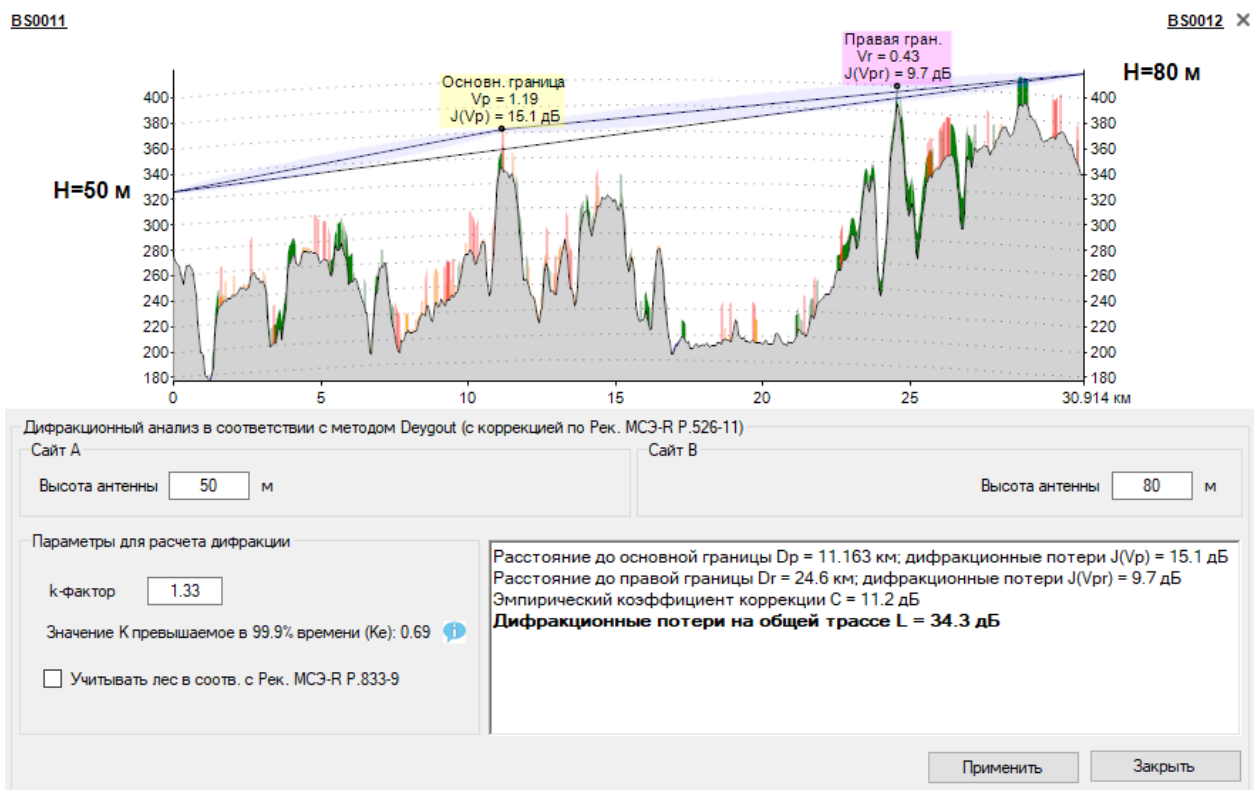
Рисунок 23. Анализ дифракционных потерь по методу Дегу по Рек. МСЭ-R P.526-11
