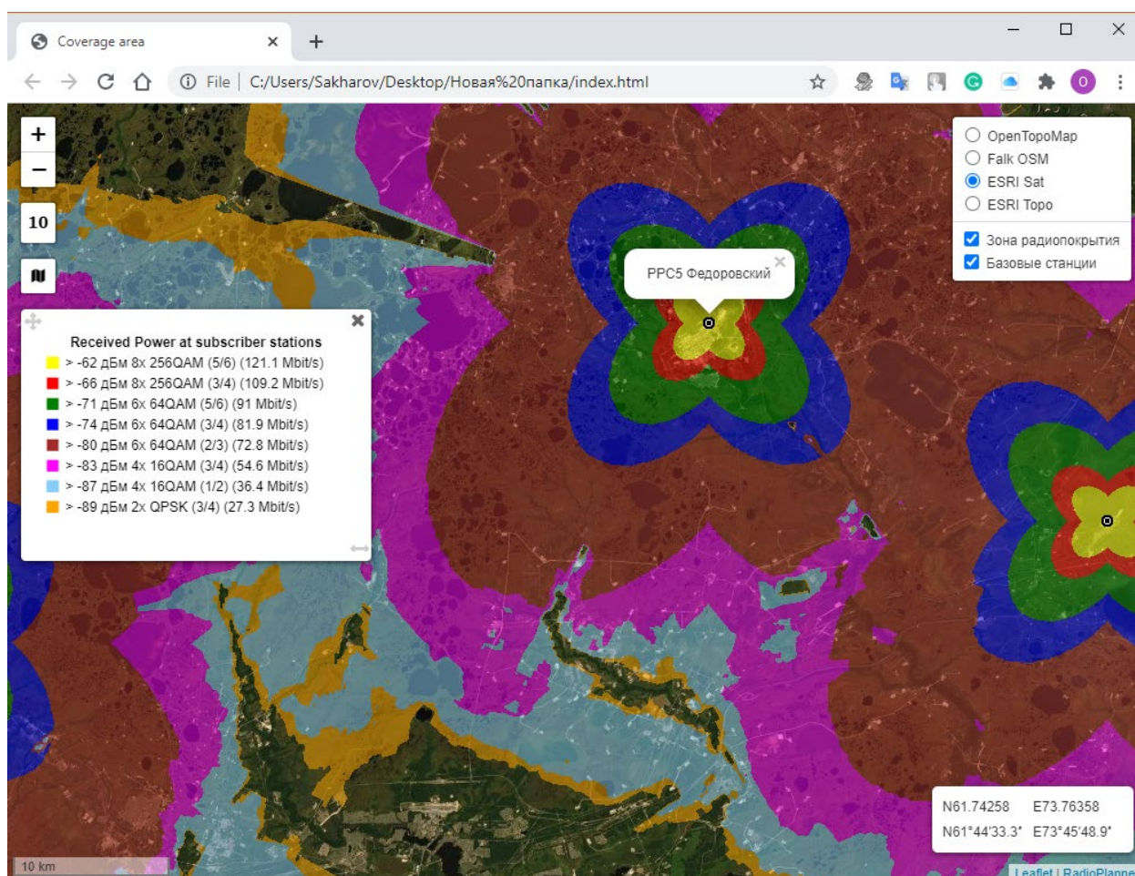
Рисунок 35. Пример результата расчетов в виде интерактивной веб-страницы
