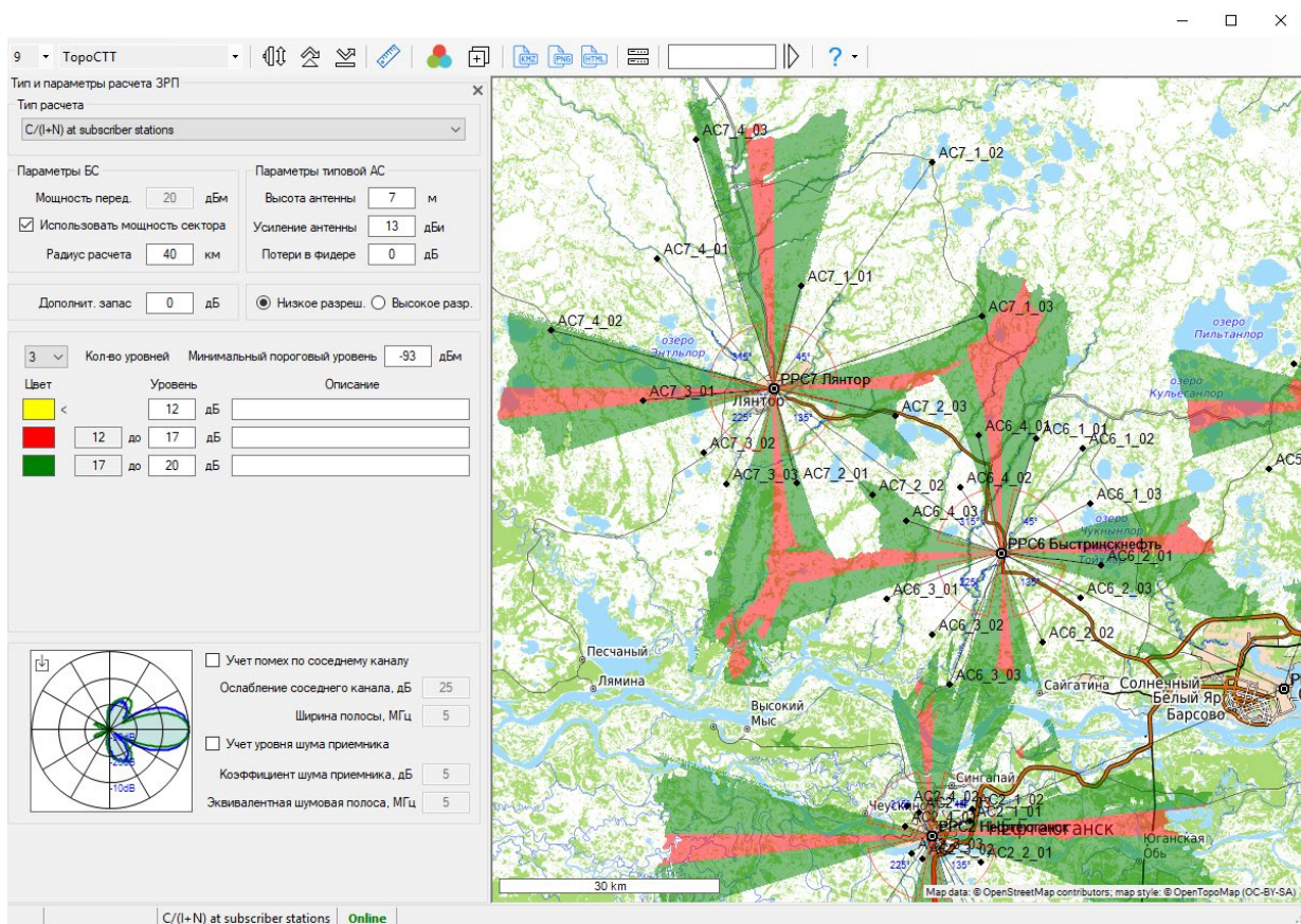
Рисунок 34. Расчет C/(I+N) на входе приемника АС
